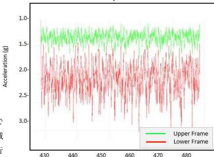
走行時の上下フレームの振動比較
